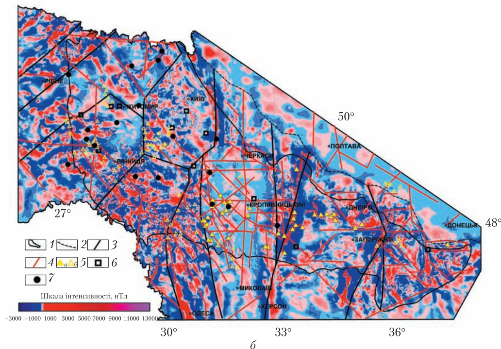
Схема зіставлення регіональної (\Delta T)_{a,рег} (а) та локальної (\Delta T)_{a,лок} (б) компонент геомагнітного поля Українського щита з аномаліями розподілу радіоактивних елементів. 1 – границя Українського щита; 2 – границя Дніпровсько-Донецького авлакогену; 3 – зони міжмегаблокових розломів; 4 – зони глибинних розломів згідно з [10, 11]; 5 – родовища (а) та прояви (б) урану [12]; 6 – родовища радонових вод; 7 – аномалії торію в кристалічних породах
